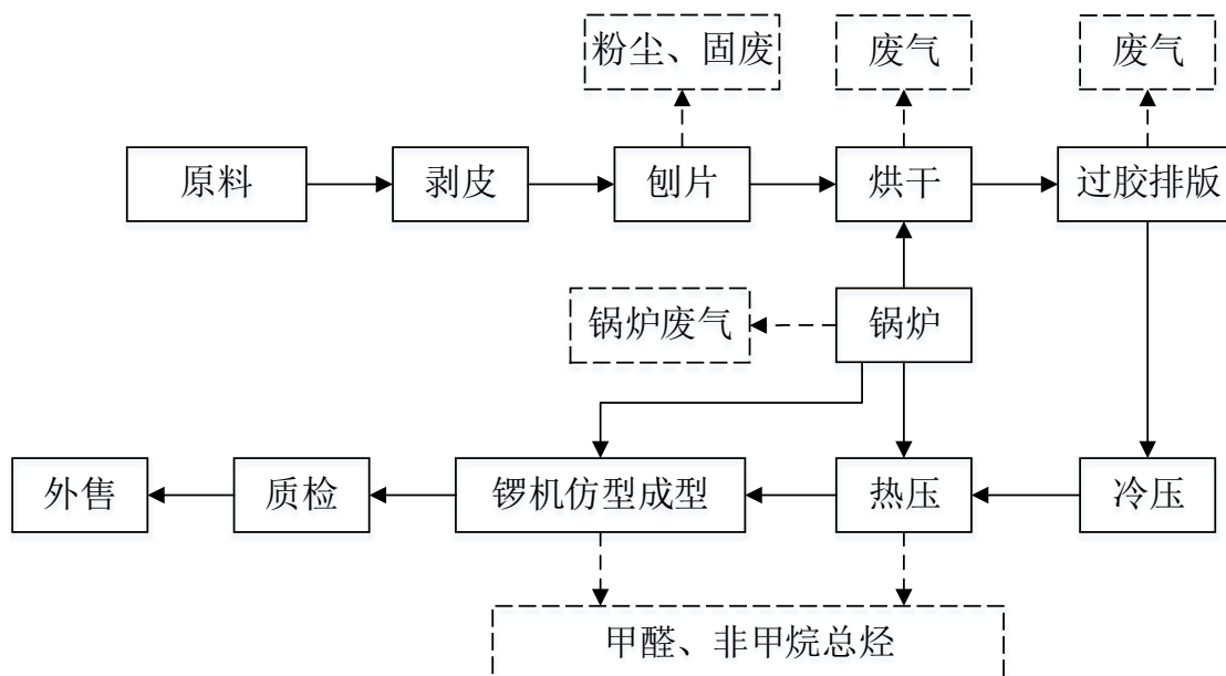
图 2-3 异型板生产工艺流程及产污环节图
